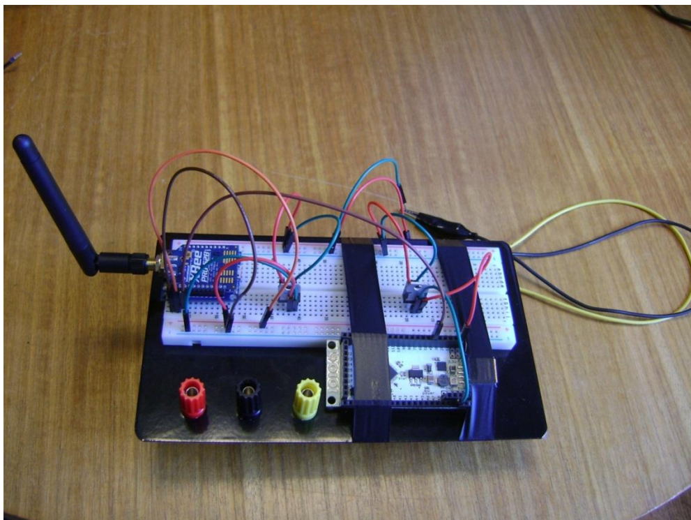
Figura 43. Módulo receptor.
