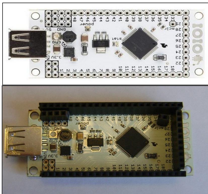
Figura 15. Placa IOIO antes y después del soldado de conectores.
