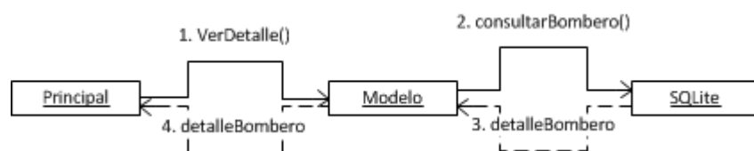
Figura 28. Diagrama de colaboración de Ver Datos.
