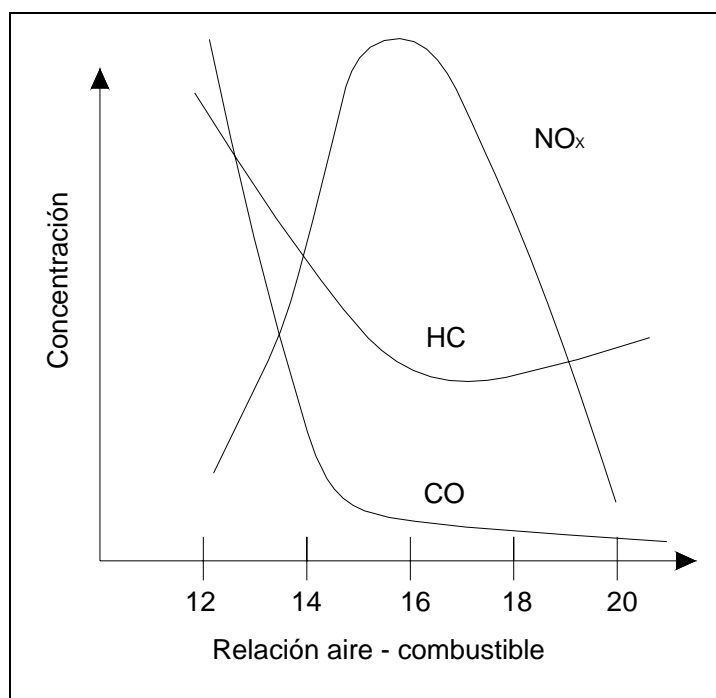
FIGURA 3-3: composición de los gases de escape en función de la relación aire – combustible (ver referencia 10 en página 90).
