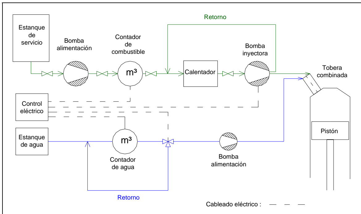
FIGURA 3-6: circuito de inyección directa de agua DWI.
