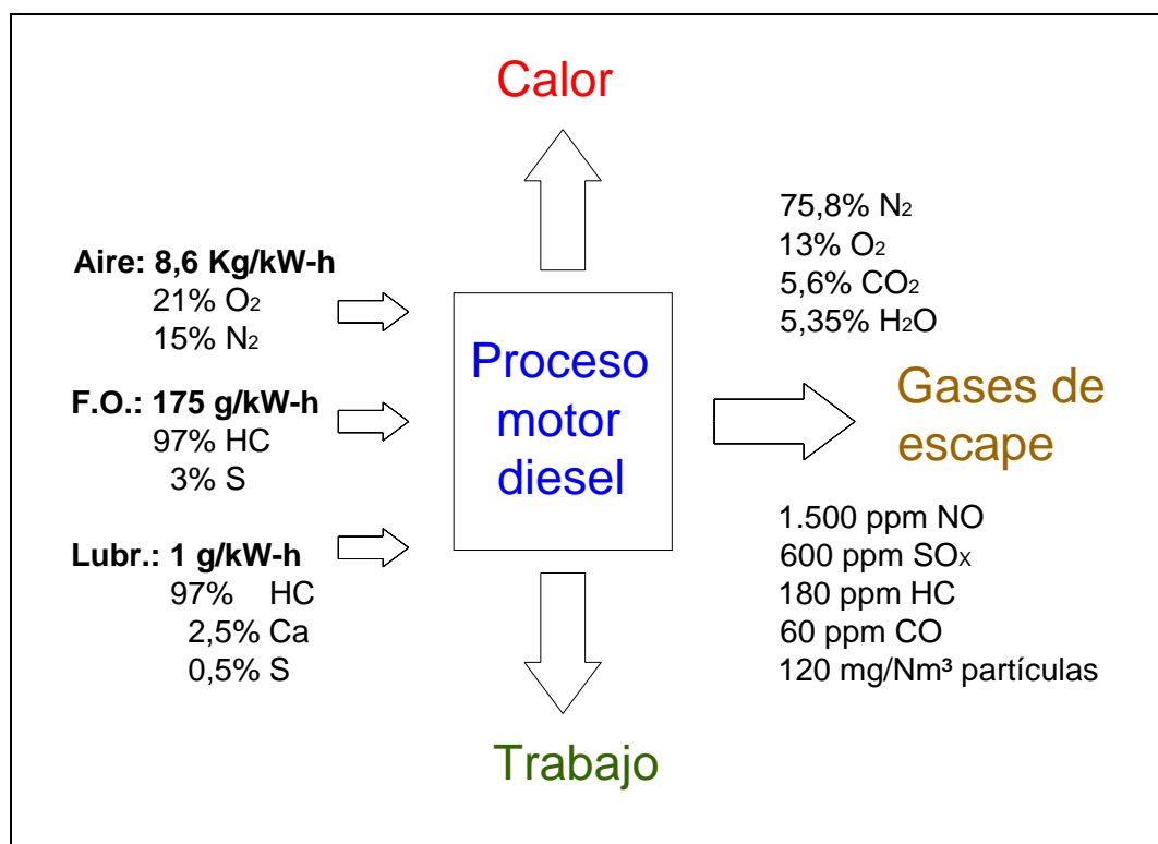
FIGURA 3-2: emisiones típicas de un motor MAN B & W diesel lento para una relación aire:combustible de 49:1, donde g/kW-h es el consumo específico del motor (ver referencia 14 en página 91).
