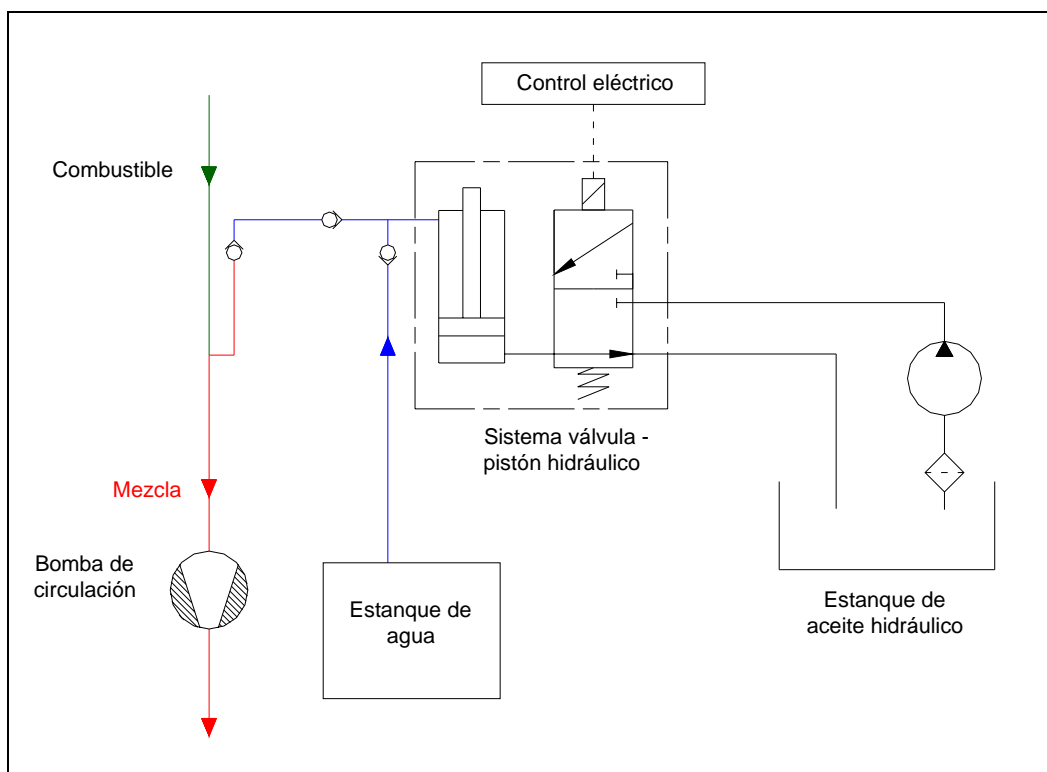
FIGURA 3-5: sistema mezclador del método SFWI (ref. 14).
