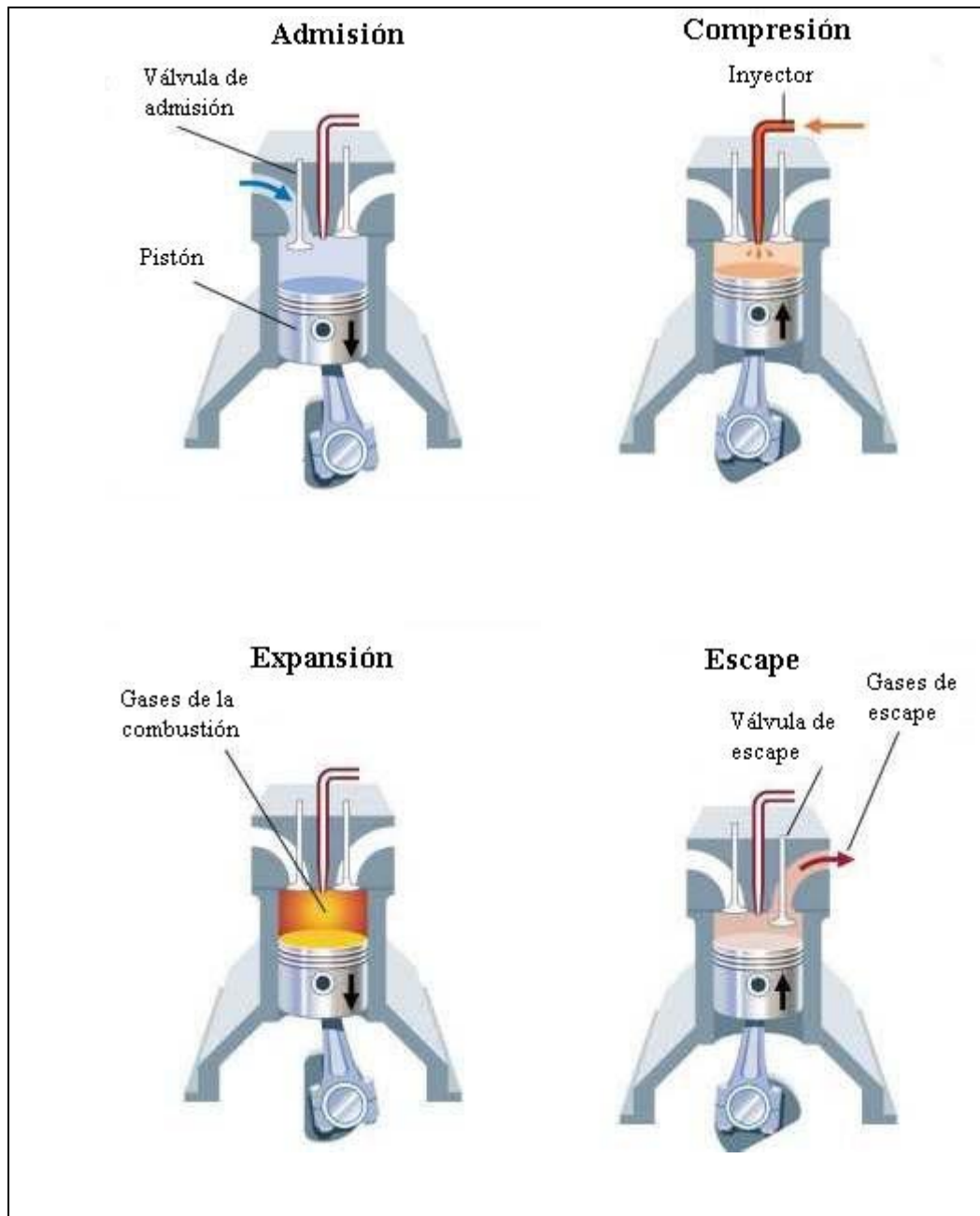
FIGURA 3-1: funcionamiento de un motor diesel marino.
