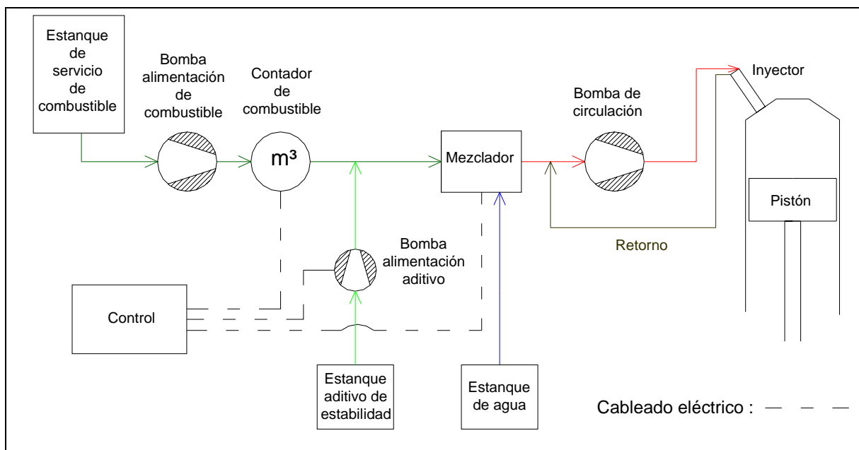
FIGURA 3-4: circuito de inyección de un combustible emulsificado con agua (ref. 14).
