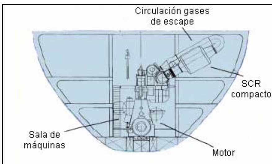
FIGURA 3-10: instalación de una unidad de reducción catalítica tipo, con respecto a su posición en un buque con motor de velocidad lenta (ref. 13).
