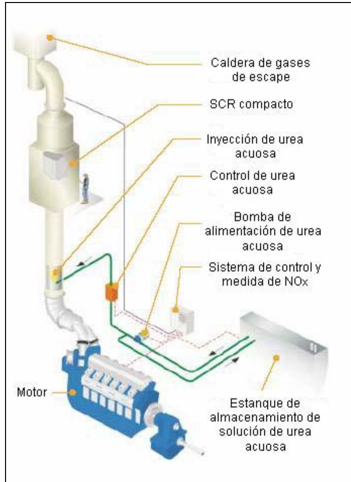
FIGURA 3-9: unidad SCR en comparación al tamaño de una persona (ref. 13).
