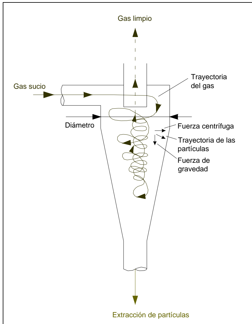
FIGURA 3-12: extracción de partículas en un multiciclón (ref. 11).
