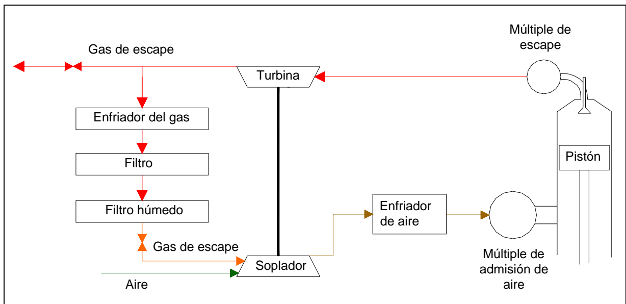
FIGURA 3-8: sistema de recirculación de los gases de escape, EGR (ref. 14).
