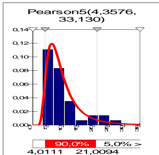
Figura 25: Distribución Arqueadura
