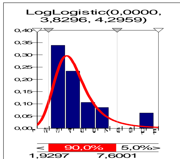
Figura 17: Distribución Encorvadura
