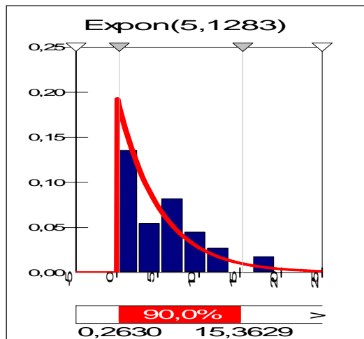
Figura 27: Distribución Torcedura
